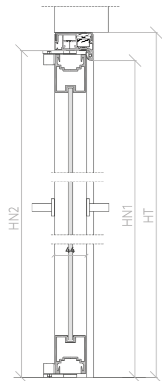
Sezione verticale Vertical section
