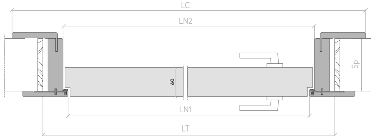
Maniglia Handle
