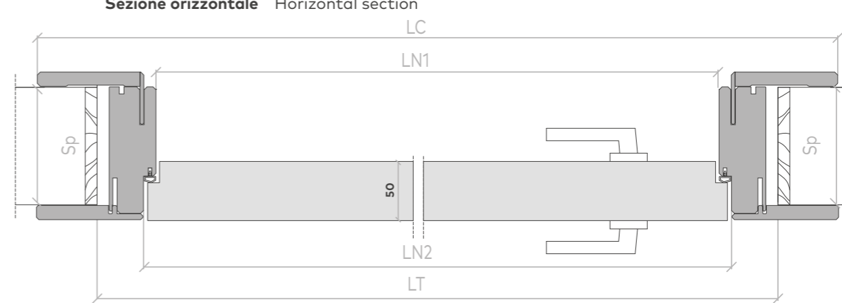
APERTURA DESTRA RIGHT OPENING
