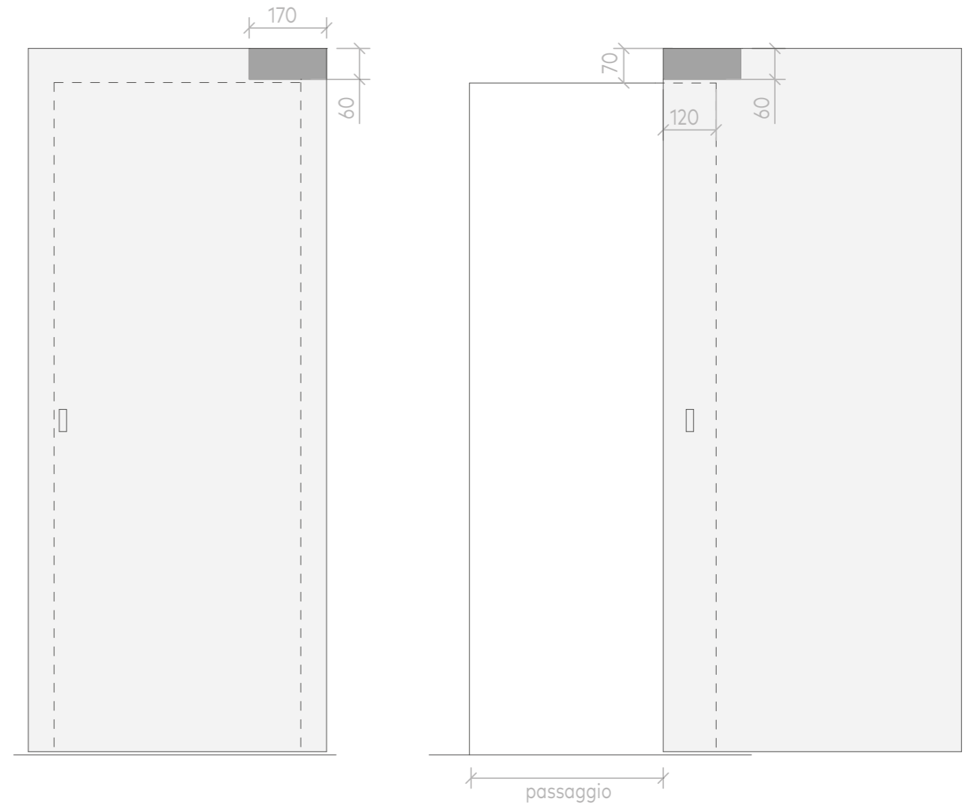
Posizione meccanismo Hardware position
