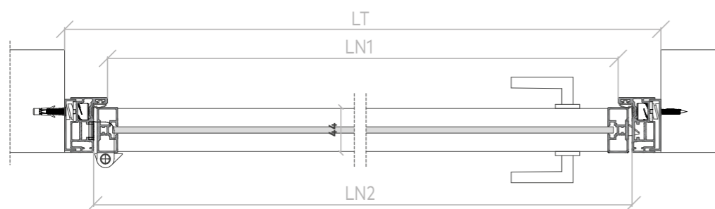
Sezione orizzontale Horizontal section
