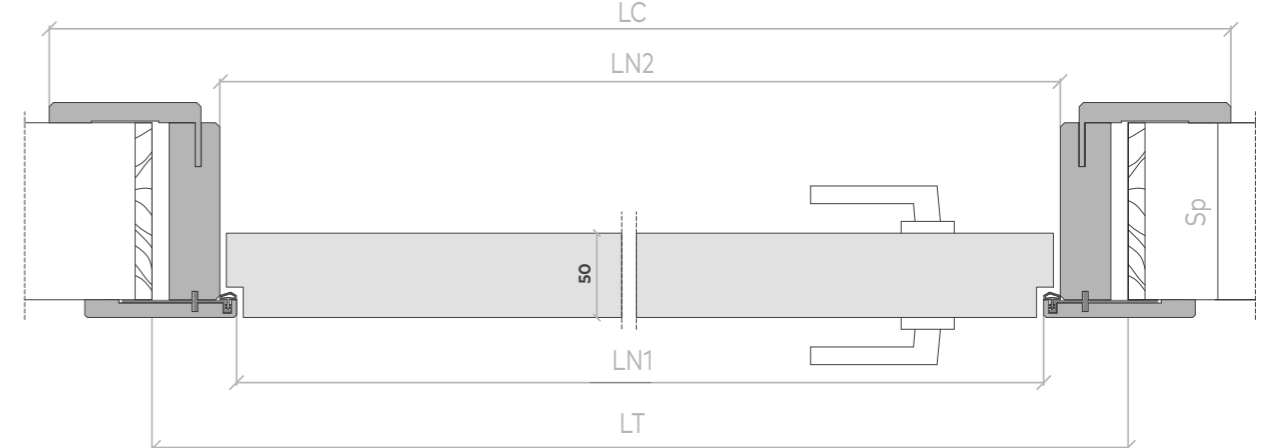
Maniglia Handle
